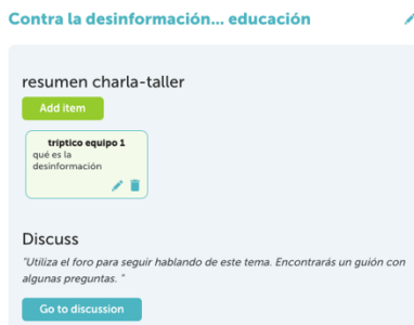
Imatge 4. TwinBoard
